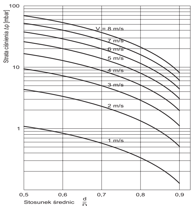
Wykres 4. Straty ciśnienia dla zwężek wg Rys. 10
