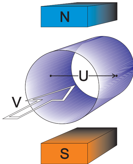
Rys. 1. Zasada działania przeływomierza elektromagnetycznego
