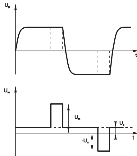
Wykres 2. Pobieranie próbek napięcia pomiarowego
